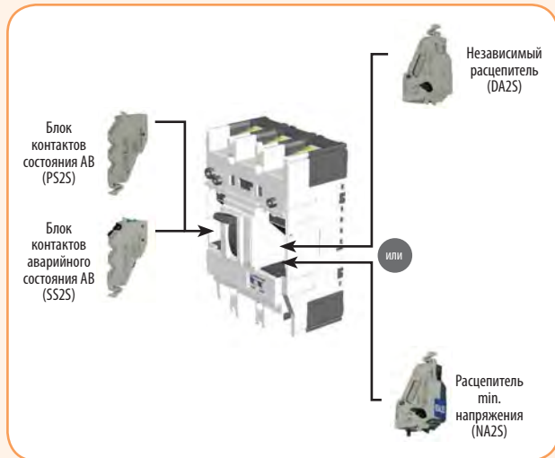
Блок контактов состояния АВ (PS2S)
