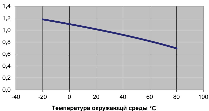
Кэффициент корреляции по температуре CH10x85 gPV 1500V DC
