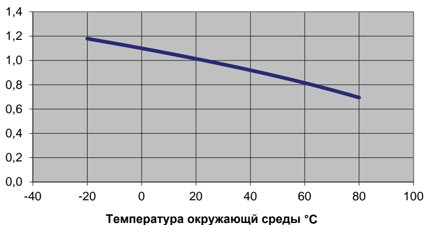
Кэффициент корреляции по температуре CH10x85 PV 1200V DC
