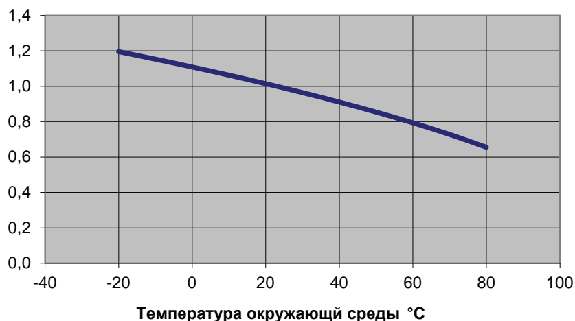
Кэффициент корреляции по температуре CH10x38 gPV 1000V DC
